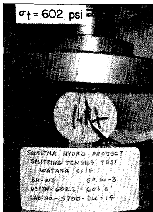
ALTERED DIORITE - TENSILE TEST
