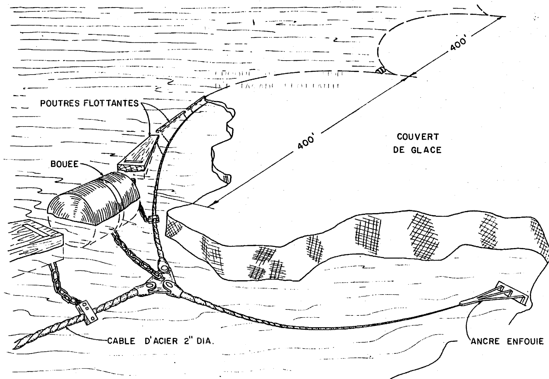
CROQUIS D'UNE SECTION D'ESTACADE FLOTTANTE
