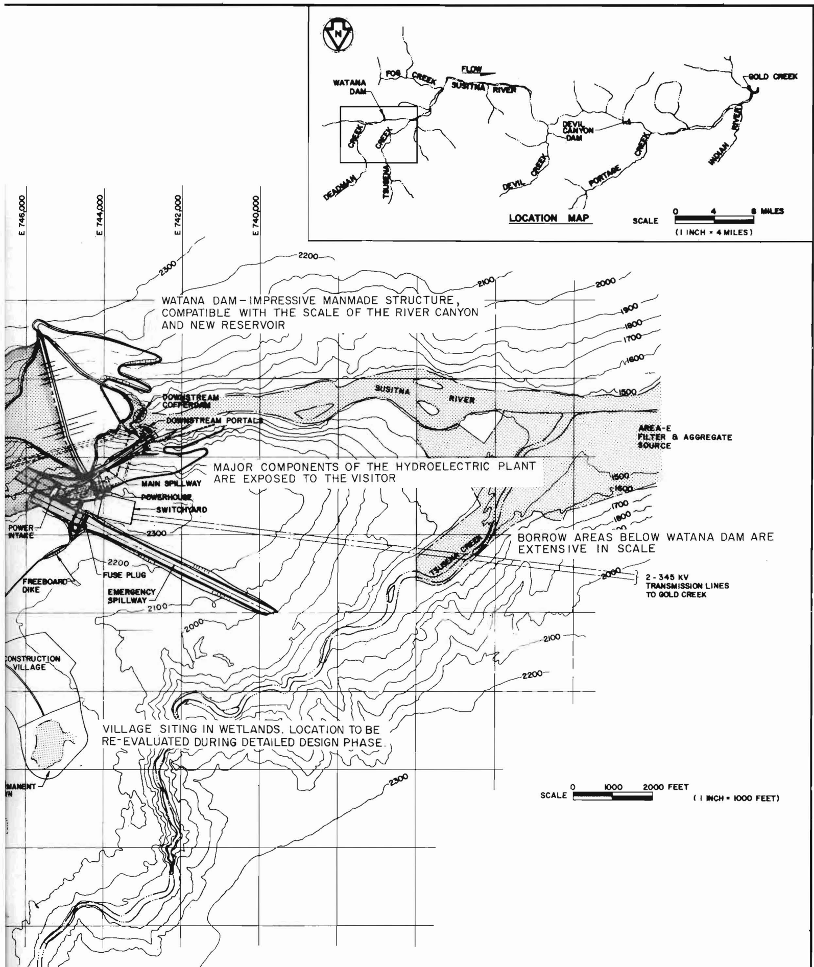
ATANA SITE LAYOUT
