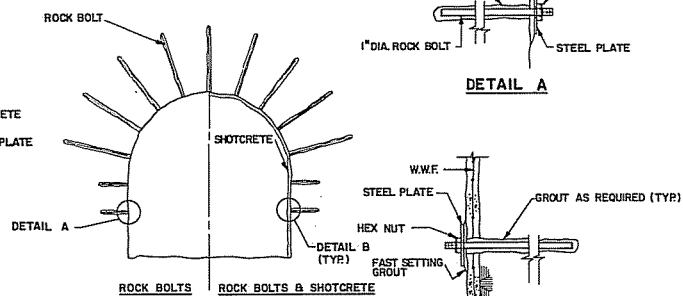
TYPICAL TUNNEL SECTIONS (N.T.S.)
