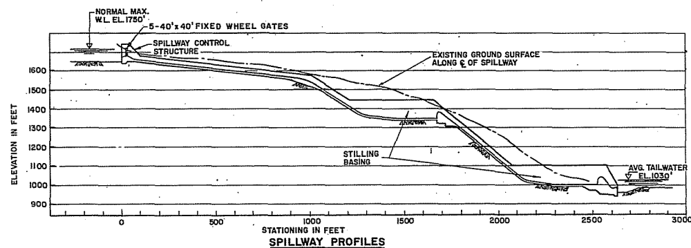
SPILLWAY PROFILES SCALE: B
