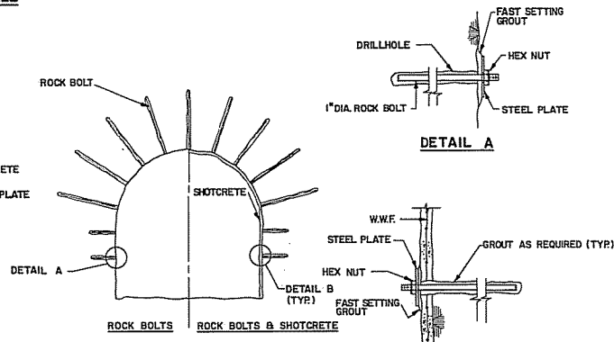
TYPICAL TUNNEL SECTIONS (N.T.S.)
