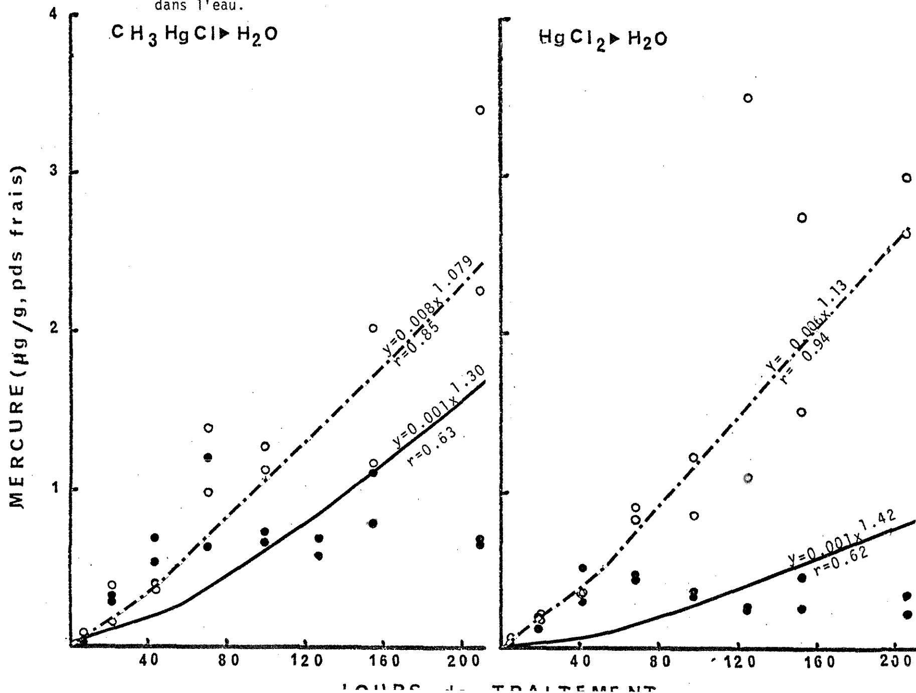
FIGURE 1. - Teneur en mercure ( \mu\text{g/g} , pds frais) mesurée dans les muscles (—) et les entrailles (0—0) des truites lors du traitement de 0.25 ppb de mercure dans l'eau.
