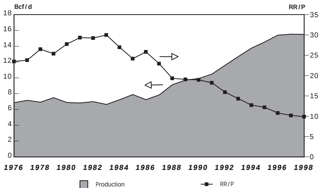
WCSB Production & RR/P
